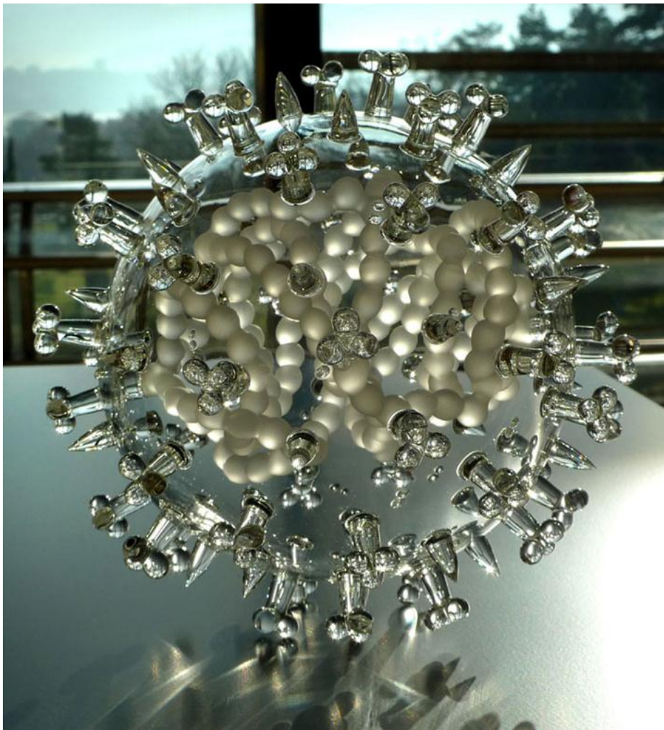
SARS Corona Virus
